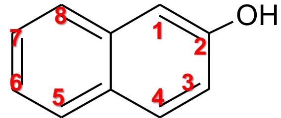
2 - hidroxinaftaleno 2 - naftol
