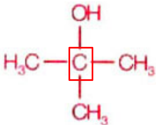
Álcool terciário
