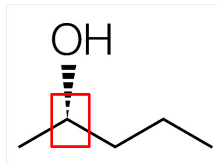
Álcool secundário
