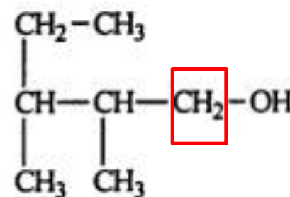
Álcool primário
