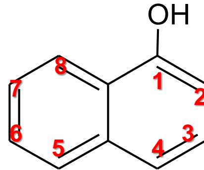
1 - hidroxinaftaleno 1 - naftol
