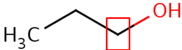
Álcool primário
