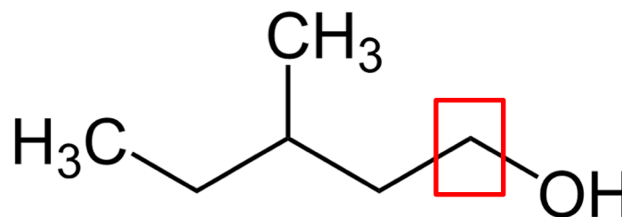
Álcool primário
